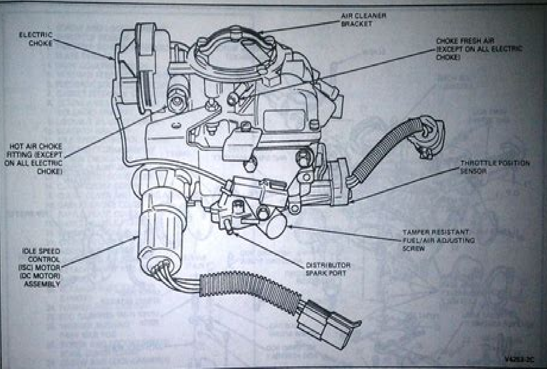
FIG. 3 YFA 1-V Feedback or Altitude Carburetor—Right Side
