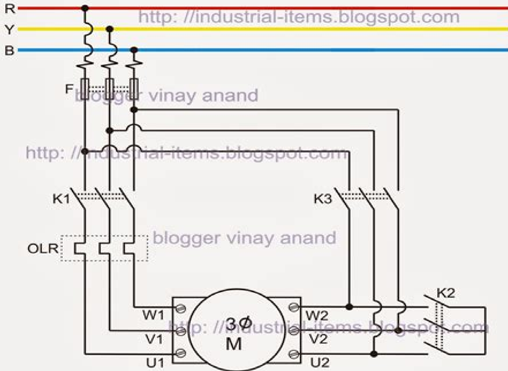
Star-Delta Motor Starter Power Ckt.
