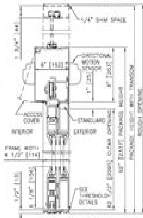
VERTICAL SECTION SCALE: 3" = 1'-0"
