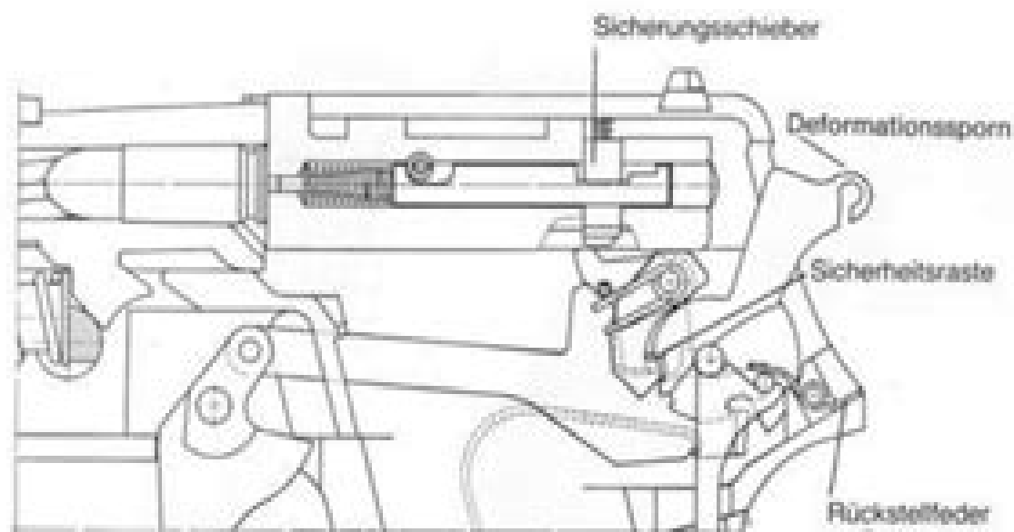
Abb. 16 Fallsicherheit
