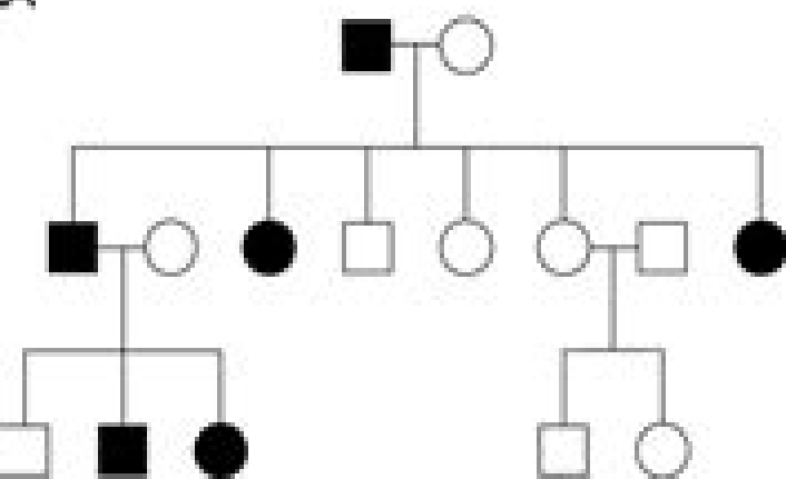
Autosomal dominant
