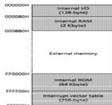
TMP93CS32 memory map
