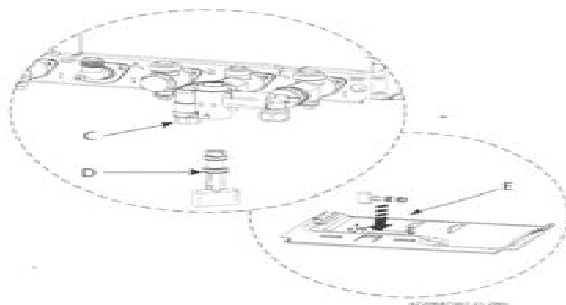
Fig. 36 Filling link key
