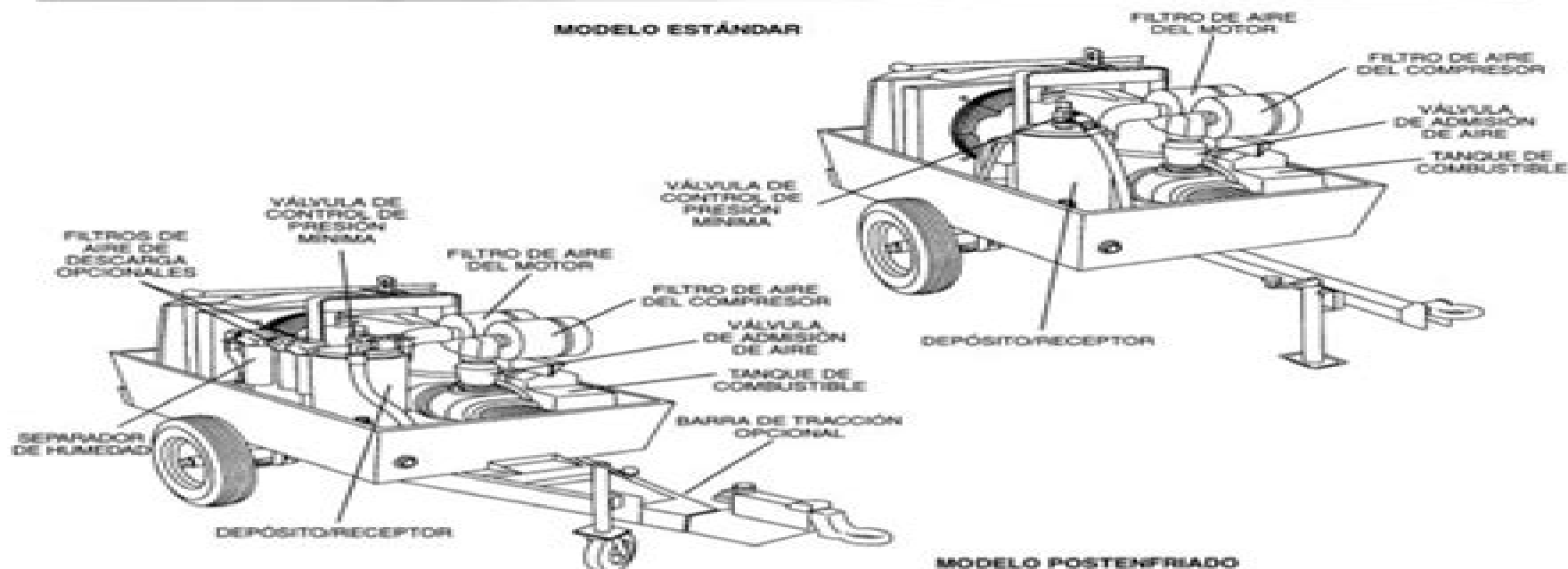
Ilustración 2-1 Compresor de Aire Portátil Sullair a Tornillo Rotativo – Modelos Estándar y Postenfriados
