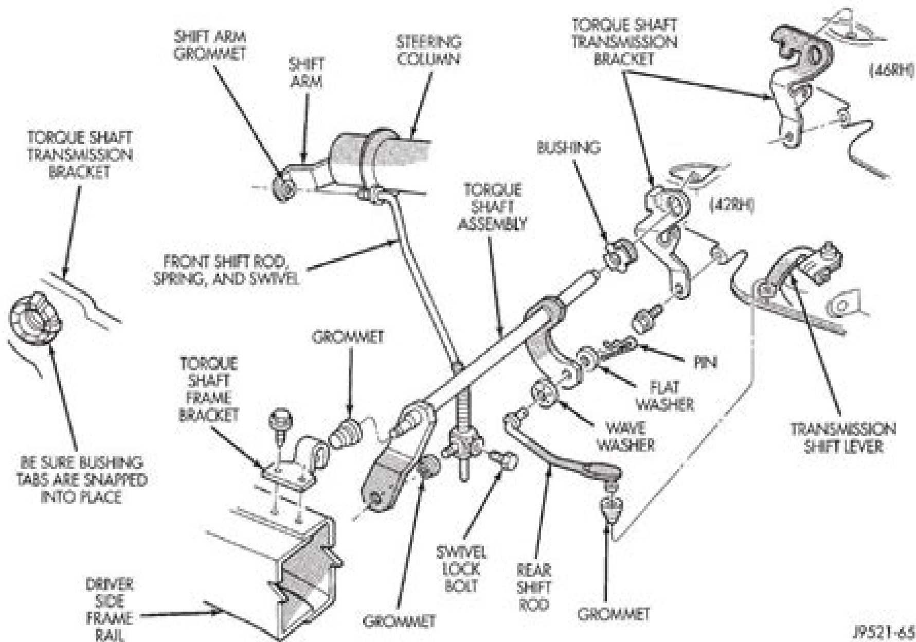
Fig. 2 Column Shift Linkage
