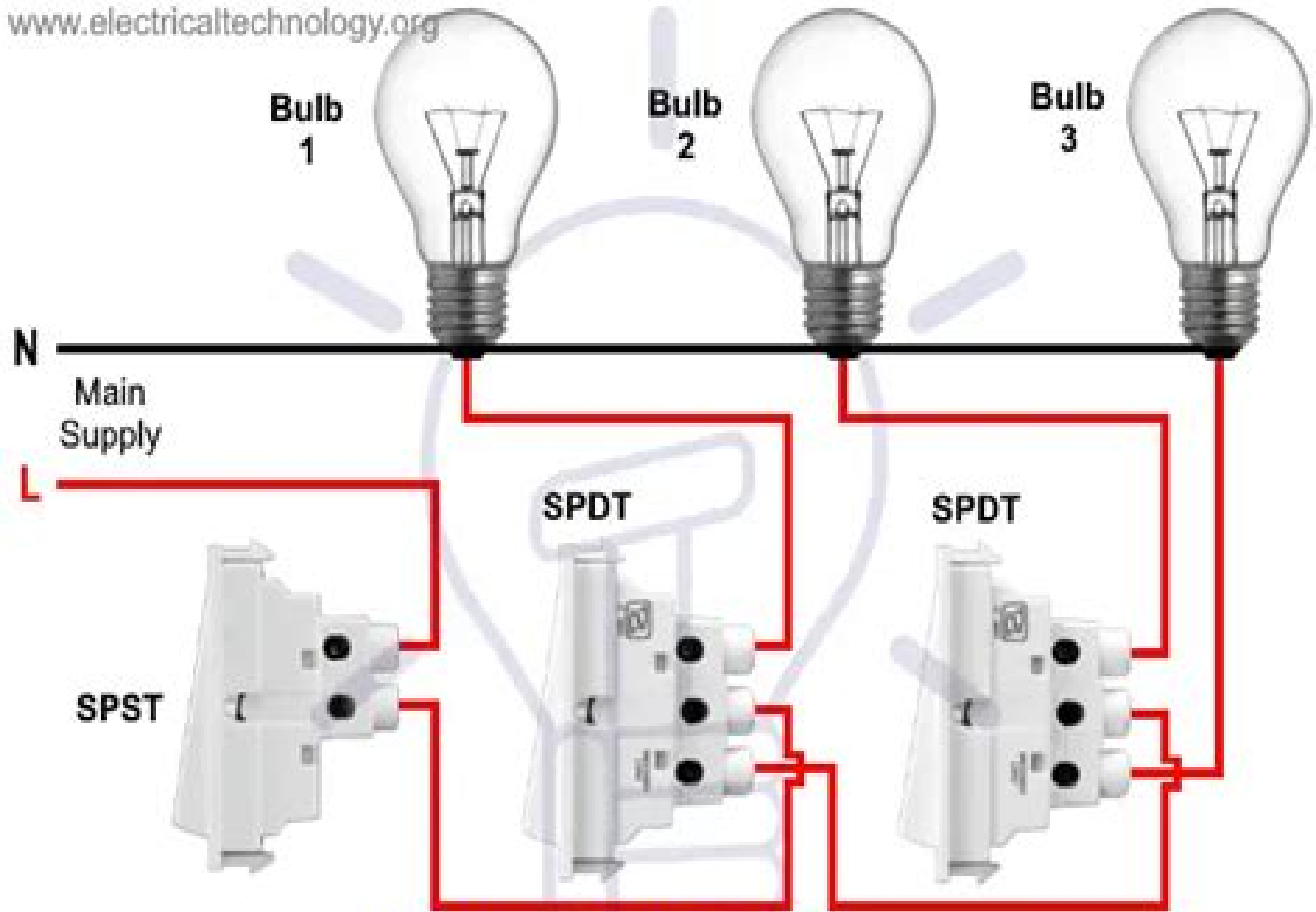
Godown Wiring Diagram
