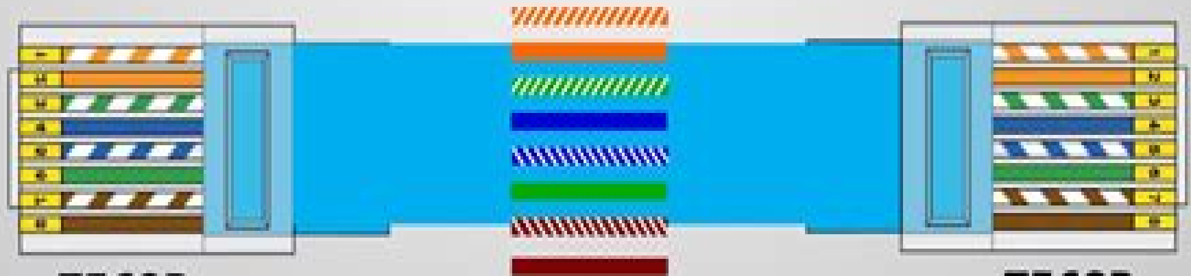
T568B
