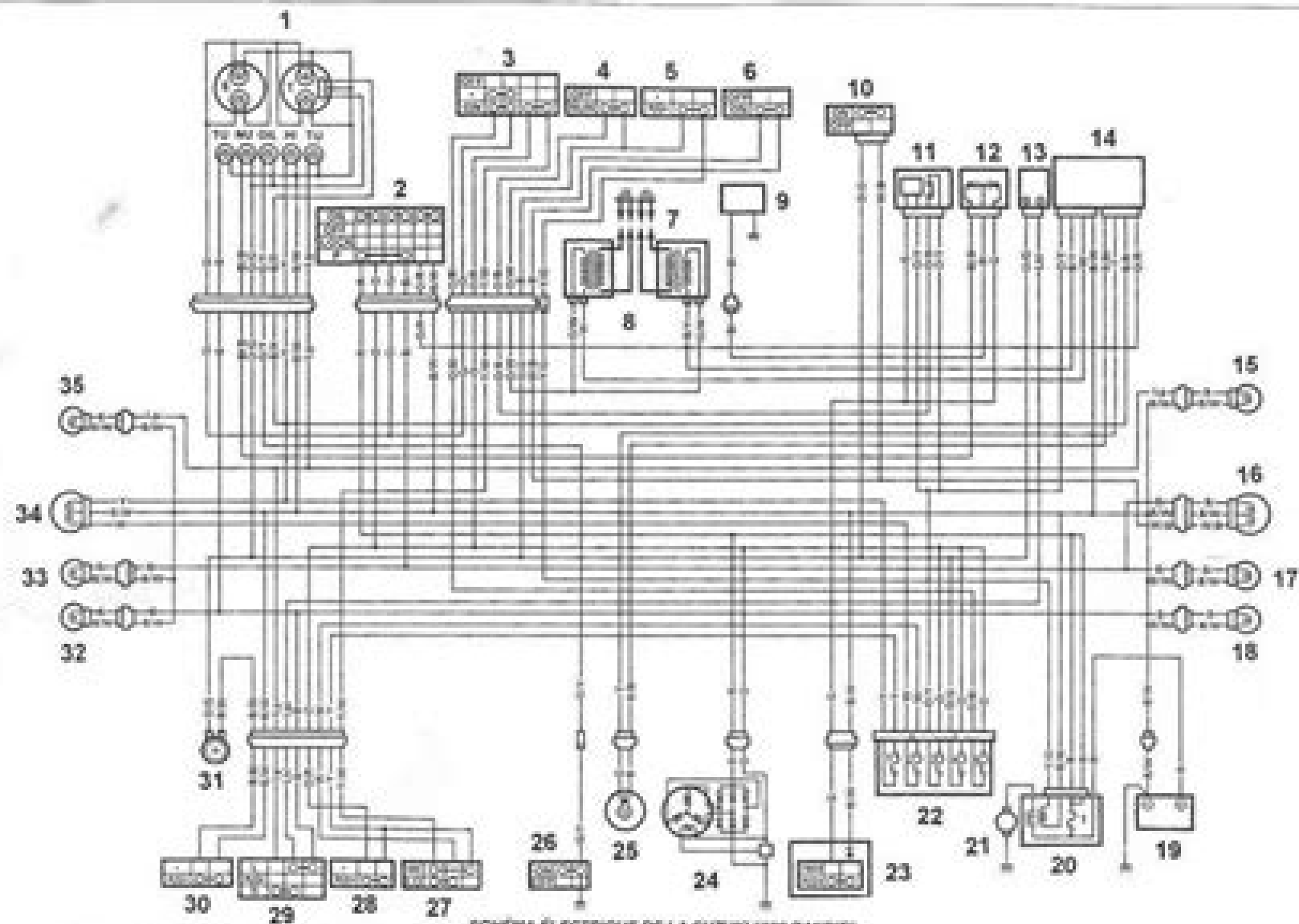
SCHEMA ÉLECTRIQUE DE LA SUZUKI "700 BANDIT"
