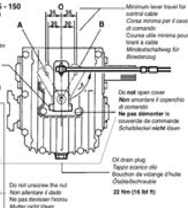
Fig. 3a Oil dipstick and filter screw, 17 mm Asta dell'olio e tappo di riempimento dell'olio (17 mm) Jauge et bouchon de remplissage d'huile (17 mm) Ölmessstab und Ölschraube SW 17
