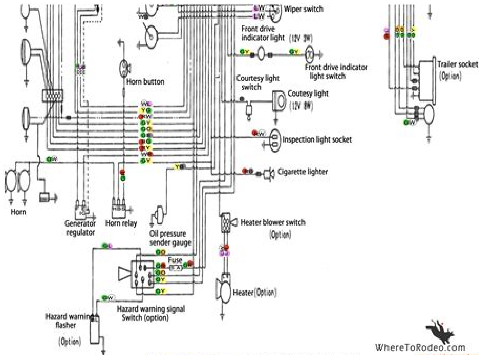
Pre-1972 Wiring Diagram (F340 (L), 45 (L), 45 (L) V, 43(L))
