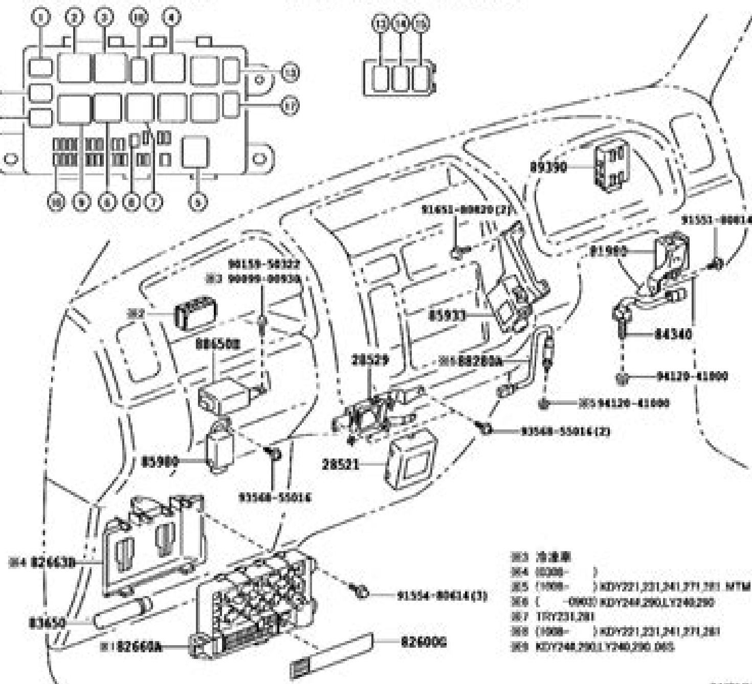
※1 カウル サイド リレーブロック
