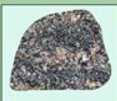
Migmatite
