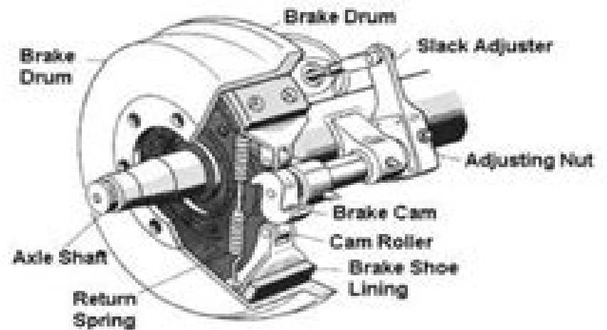
Air Brake
