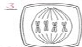
Metaphase
