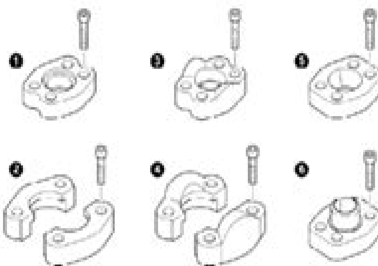
Fig. 1 SAE flanges
