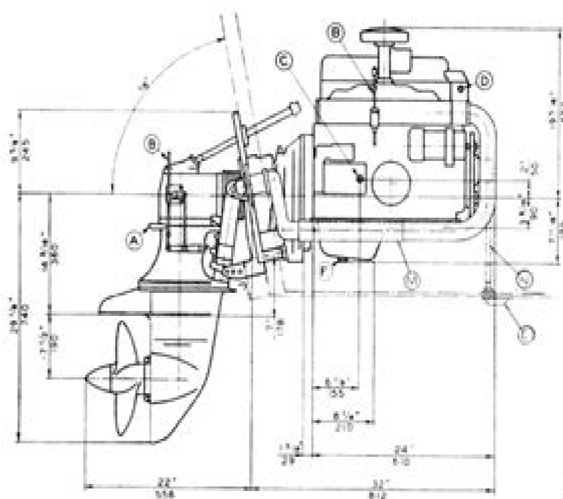
Volvo Penta AQ80/100 Masszeichnung
