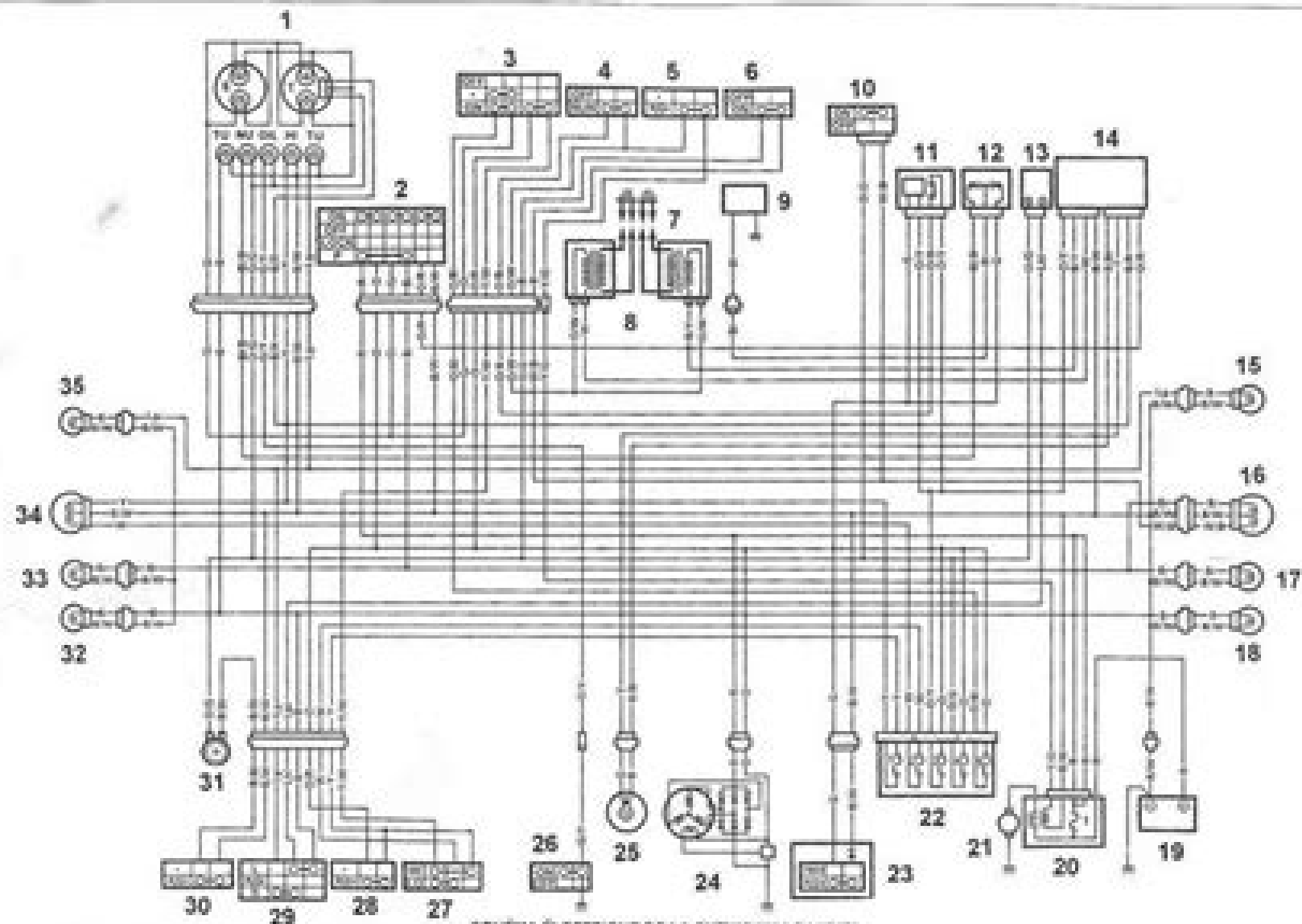
SCHEMA ÉLECTRIQUE DE LA SUZUKI "800 BANDIT"
