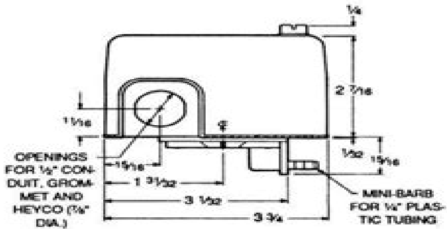
69ES with 90° Mini Barb Dimensions
