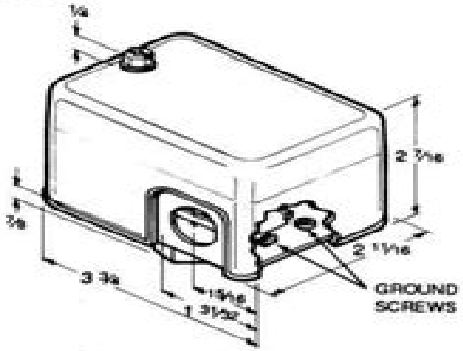
69ES Dimensions
