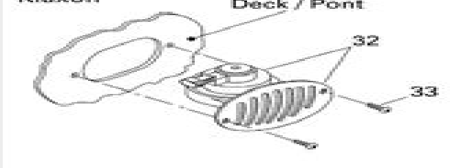
Horn / Klaxon
