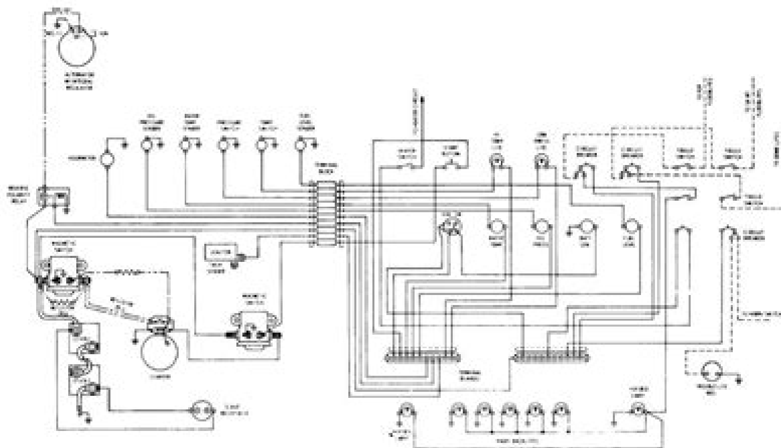
图 10-10 机床电气控制线路图
