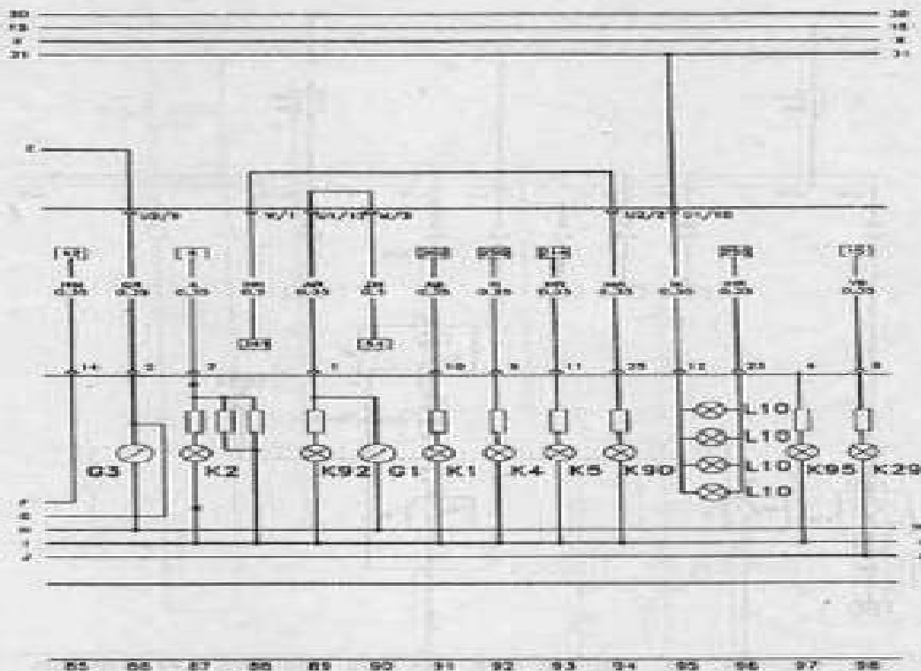
Схема 6: Приборы, сигнальные лампы, индикатор топлива
