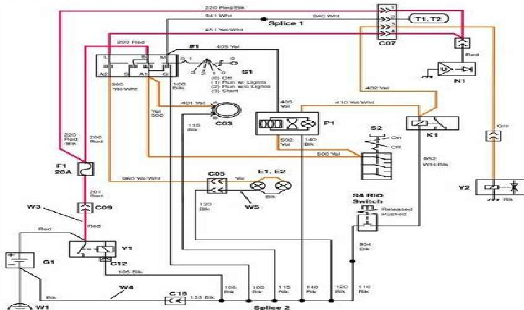
D140, D150, D155, D160, D170 Power Circuit Schematic
