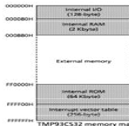
TMP93CS32 memory map
