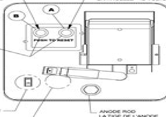
ECO SWITCH & T-STAT 12V DC: SPARK IGNITION INTERRUPTEUR ET THERMOSTAT ECO - ALLUMAGE PAR ENTROUVERTE - 12 VOLTS DC
