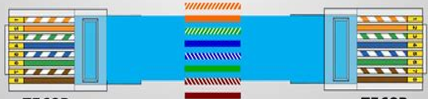
T568B
