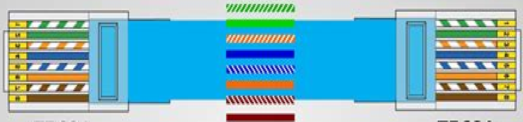
T568A
