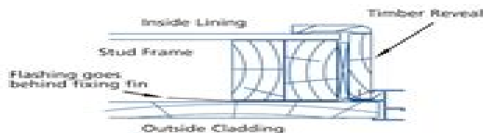
TIMBER FRAME JAMB
