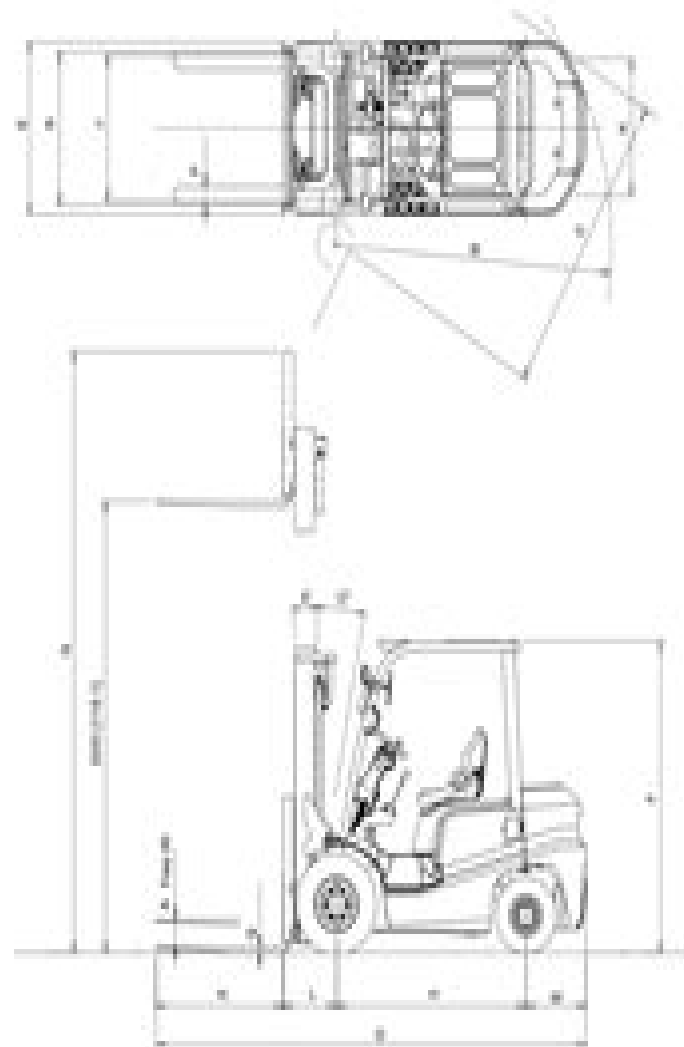
Fig. 1 Fork Dimensions
