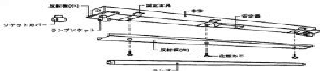
■ 単体用ソケットカバー(別表)の仕様
